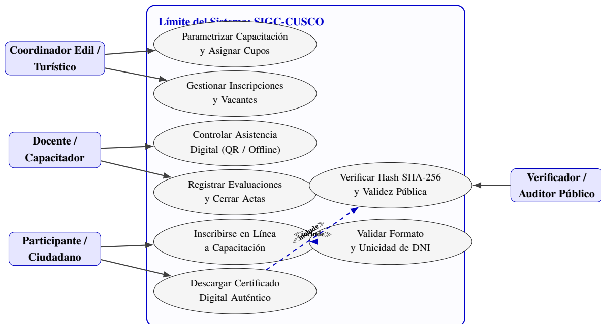
Figura 1: Diagrama de Casos de Uso del Sistema SIGC-CUSCO con delimitación de frontera funcional.
