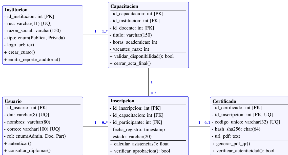
Figura 2: Diagrama de Clases del Dominio con atributos, métodos y cardinalidades normalizadas.
