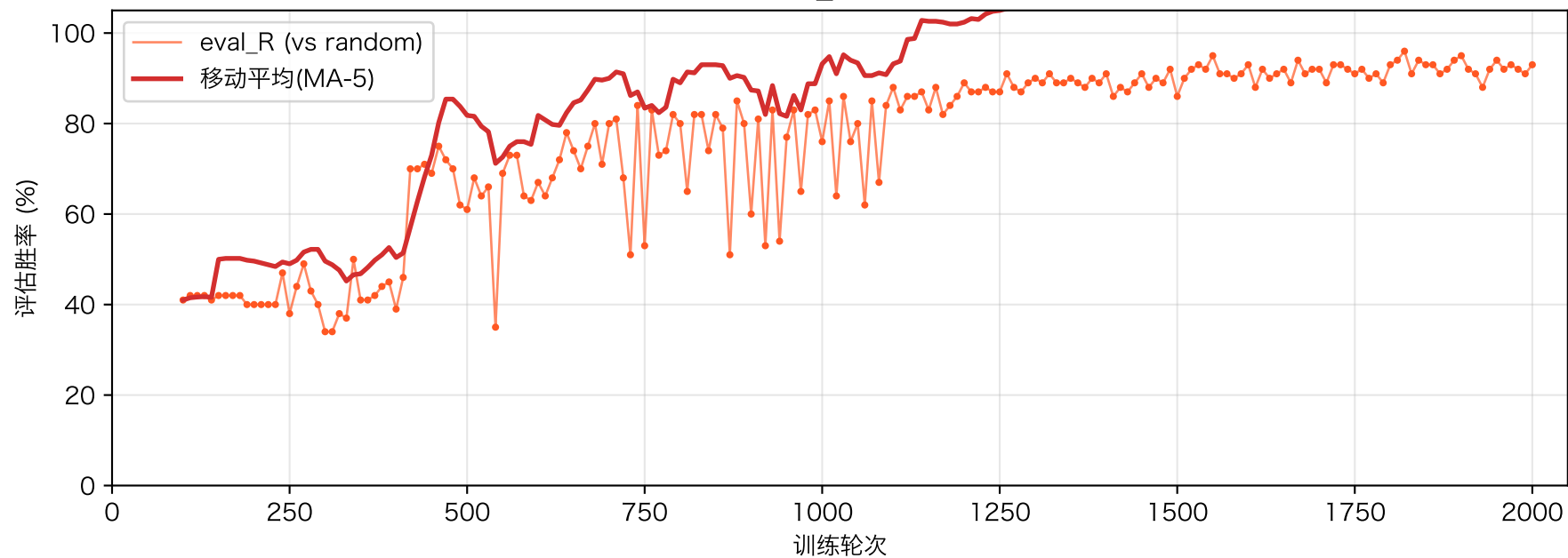
v49 eval_R 变化曲线
