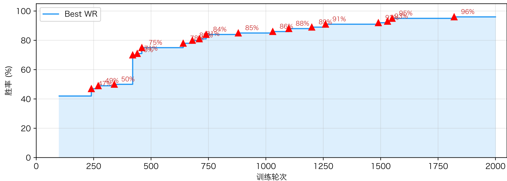
v49 Best WR 变化曲线
