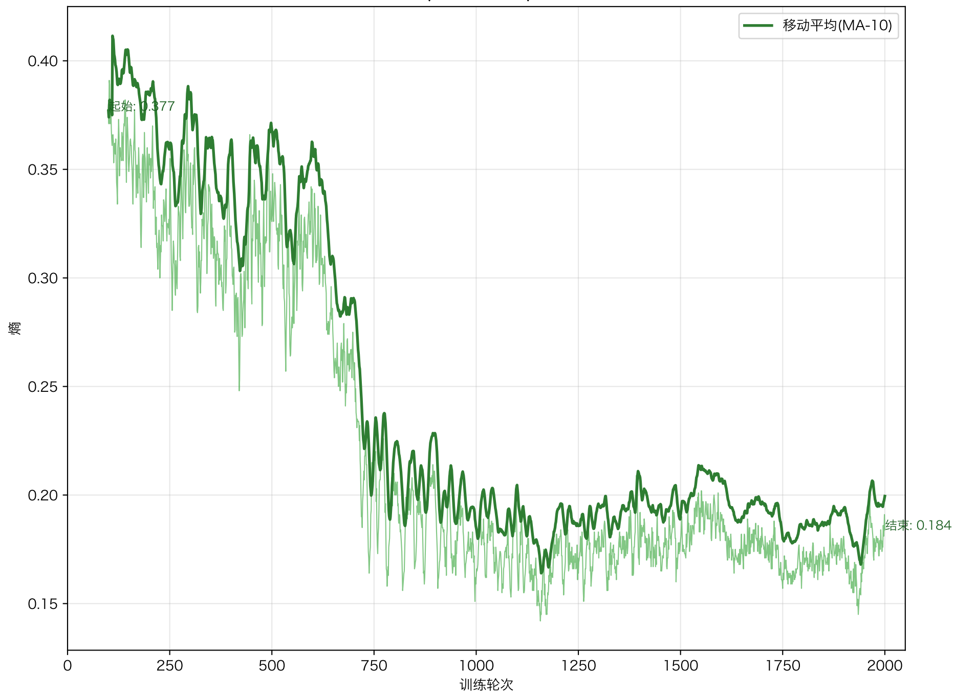
v49 熵 (策略探索度) 变化曲线
