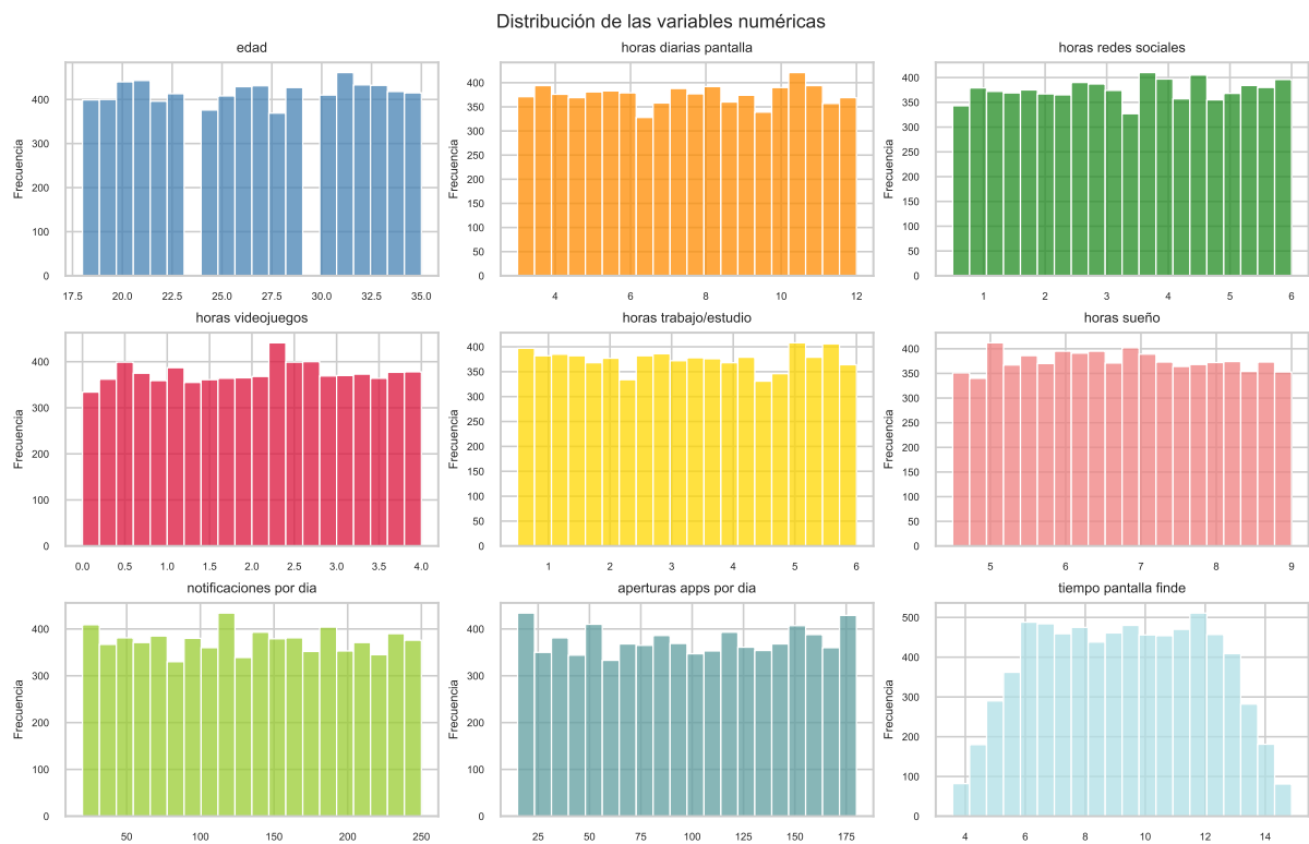
Figura 2: Histogramas de las variables numéricas del dataset.
