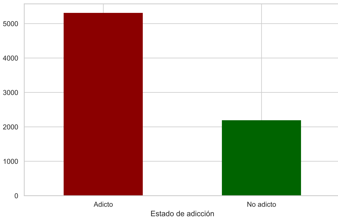
Figura 1: Distribución de la variable objetivo: estado de adicción (0 = No adicción, 1 = Con adicción).
