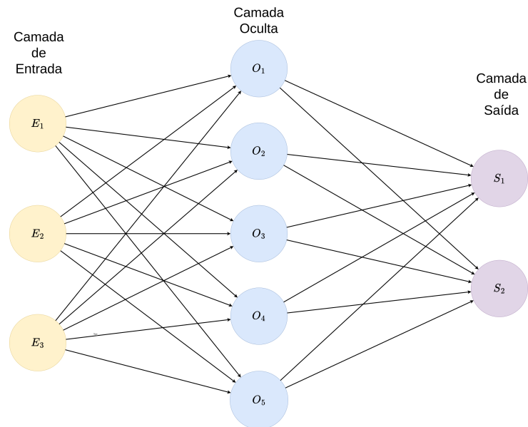
Figura 2.2: Arquitetura de uma rede neural básica
