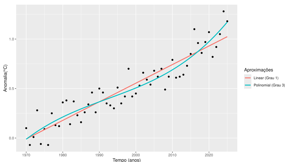
Figura 2.1: Gráfico da anomalia ( ^{\circ}\text{C} ) em função do tempo (anos), 1970-2025, com regressão linear, e polinomial de grau 3
