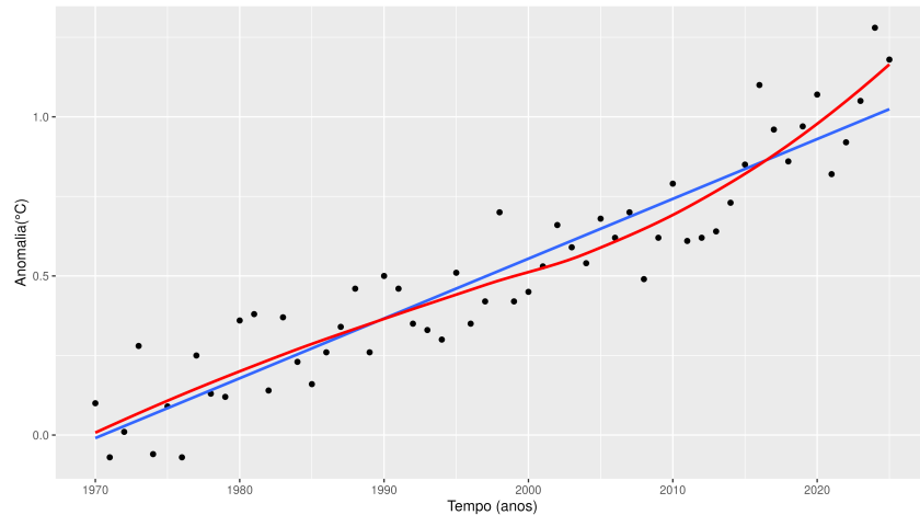
Figura 2.3: Gráfico da anomalia (°C) em função do tempo (anos), 1970-2025, com regressão linear e aproximação polinomial
