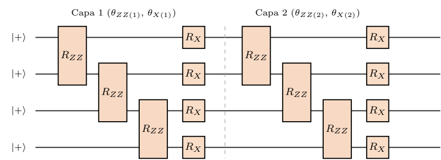
Representacion de circuito HVA. Cada R_{ZZ} se descompone como CX \cdot R_Z \cdot CX (2 compuertas de dos qubits por termino). El orden de aplicacion es de izquierda a derecha.
