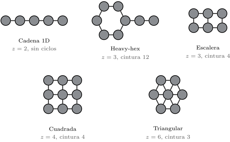
Topologías ordenadas por número de coordinación z creciente.
