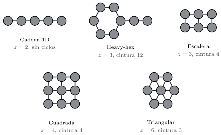
Topologias ordenadas por numero de coordinacion z creciente.
