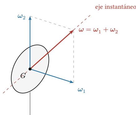
Figura 1: El disco de la horquilla, ya visto en el módulo 18 (allá, para hallar \omega ; acá, para hallar H_G ). Los ejes \hat{i}, \hat{j}, \hat{k} , clavados a la horquilla, son en todo instante ejes principales del disco: \hat{k} es su eje de simetría y \hat{i}, \hat{j} son diámetros.
