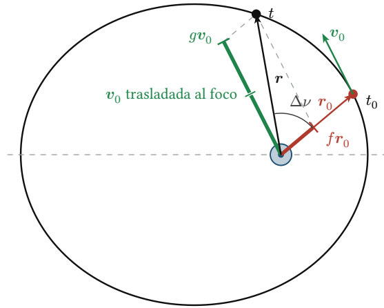
Figura 2: Por qué los coeficientes de Lagrange tienen que existir. Lo que hay que sacar del dibujo es que la posición nueva r es la diagonal de un paralelogramo cuyos dos lados están sobre los dos vectores que ya se conocían, y que el único paso conceptual del asunto es tener que trasladar v_0 al foco para poder dibujar el segundo lado: ahí v_0 deja de ser la velocidad de alguien y pasa a ser el vector de una base. Con los valores de la figura, f = 0,45 y g = 1,87 .
