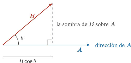
Figura 1: La proyección de \mathbf{B} sobre \mathbf{A} . El producto escalar mide el largo de esa sombra, multiplicado por |\mathbf{A}| .
