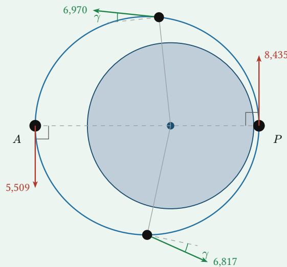
Figura 3: El satélite del ejercicio, redibujado con los datos de la figura de la cátedra. En los ápsides v es perpendicular al radio; en las dos posiciones intermedias forma un ángulo \gamma con esa perpendicular. Velocidades en km/s.
