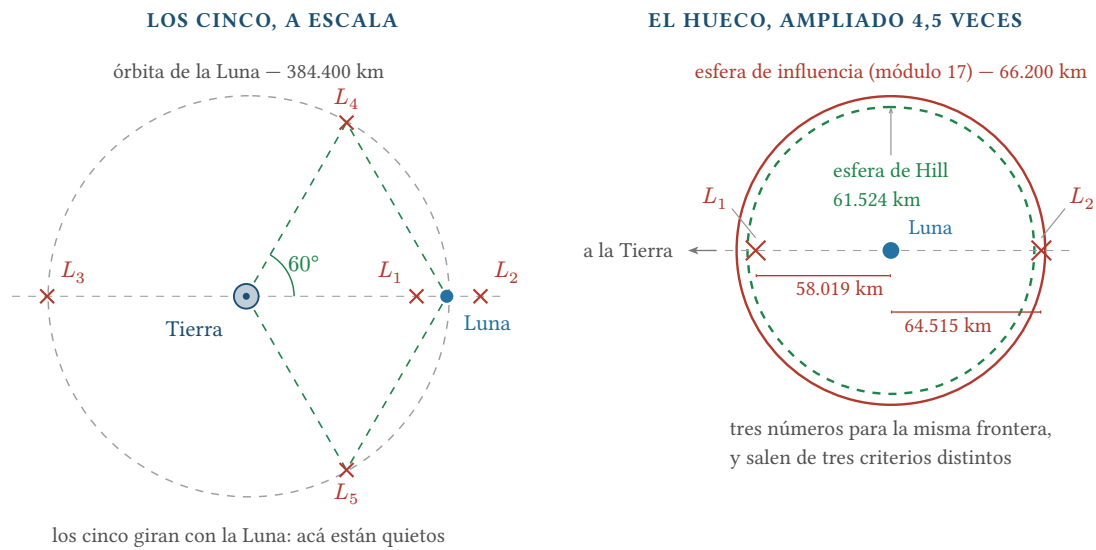
Figura 2: Los cinco puntos de Lagrange del par Tierra-Luna. En el panel (a), a escala real: L_4 y L_5 están sobre la propia órbita de la Luna, 60° por delante y por detrás, formando con la Tierra y la Luna dos triángulos equiláteros —eso es la ec. (14) dibujada—, y los tres colineales caen sobre el eje, con L_3 casi en el punto opuesto a la Luna. El panel (b) amplía la zona que el panel (a) no puede mostrar: L_1 y L_2 están a menos de 65 000 km de la Luna, y ahí aparecen tres fronteras que miden lo mismo y no coinciden — las dos distancias a L_1 y L_2 , la esfera de Hill de la sección que sigue, y la esfera de influencia del módulo 14. Entre la más chica y la más grande hay un 14%, y la sección que sigue mide esa diferencia y explica de dónde sale.
