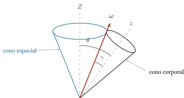
Figura 1: Los dos conos del módulo 18, reusados: tangencia externa , el corporal como un cono aparte que toca al espacial desde afuera a lo largo de \omega . Es la configuración de un cuerpo achatado — I' > I — y de la precesión directa: el Problema 4 de abajo es un caso así.
