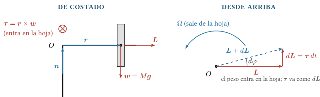
Figura 1: El giróscopo apoyado en un pivote. De costado: el peso hace un torque \tau = r \times w horizontal, que entra en la hoja. Desde arriba: ese torque le suma a L un dL perpendicular, y el eje gira un ángulo d\varphi sin cambiar de largo. Redibujada de S&Z Figs. 10.34 y 10.35, pág. 323–324.
