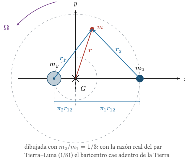
Figura 1: El marco que gira con los dos cuerpos, que es el cambio de punto de vista del que sale todo el módulo. Lo que hay que sacar del dibujo son tres cosas: que el origen es el baricentro G y no el cuerpo grande; que en este marco m_1 y m_2 están clavados sobre el eje x , cada uno a su fracción de la distancia r_{12} ; y que la nave se ubica con tres vectores distintos -r desde G , r_1 desde m_1 y r_2 desde m_2 — porque las tres cosas que hay que calcular se miden desde tres lugares distintos. La flecha curva \Omega es lo único que recuerda que el marco entero está girando.
