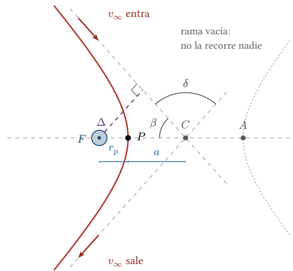
Figura 1: La hipérbola y todo lo que se le mide. El cuerpo central está en el foco F y la nave recorre la rama de la izquierda: entra desde el infinito por una asintota, dobla alrededor de F pasando por el perigeo P , y se va por la otra. La rama punteada de la derecha es la imagen matemática de la ecuación —haría falta una gravedad que empujara en vez de atraer, así que no la recorre nadie—, pero su vértice A es lo que la fórmula del apogeo devuelve, y por eso aparece. El centro C es el punto medio entre P y A : el semieje a se mide desde ahí, no desde el foco . El ángulo \beta es el que las asintotas forman con la línea de ápsides, \delta es lo que se tuerce la velocidad de punta a punta, y \Delta —el radio de puntería— es la distancia entre la asintota de entrada y una paralela que pase por F : es la puntería con la que hay que apuntar desde lejos.
