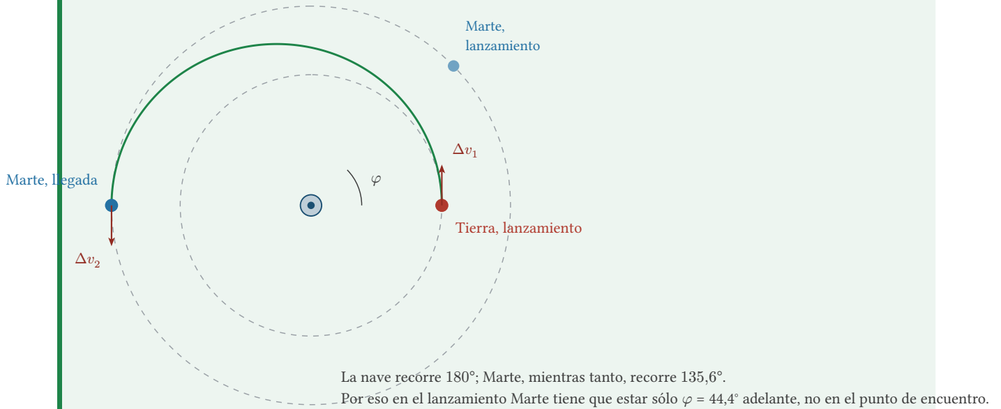
Figura 1: La transferencia de Hohmann Tierra-Marte (a escala aproximada de radios). La nave recorre 180^\circ en 258,8 días; Marte, mientras tanto, recorre 135,6^\circ de su propia órbita — por eso en el lanzamiento tiene que estar apenas 44,4^\circ adelante de la Tierra, no en el punto de encuentro.
