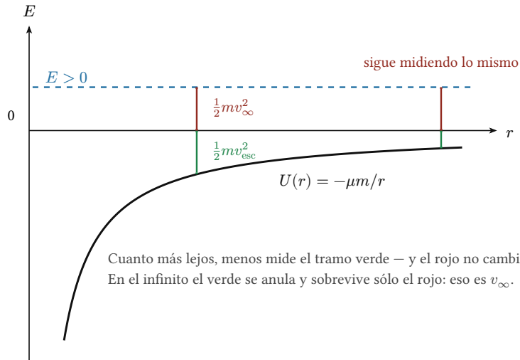
Figura 2: Por qué a la hipérbola le sobra velocidad. Es el pozo de potencial del módulo 6 con una sola recta de energía, la del caso E > 0 . A cualquier distancia r , la energía cinética es la distancia vertical entre la recta y la curva: el tramo verde es lo que se gasta en salir del pozo —justo \frac{1}{2}mv_{\text{esc}}^2 — y el rojo es lo que queda por encima del cero. A medida que r crece el tramo verde se achica y el rojo no cambia , porque la recta de energía es horizontal. En el infinito el verde vale cero y sólo queda el rojo: ésa es la energía cinética con la que la nave llega, y su velocidad es v_{\infty} .
