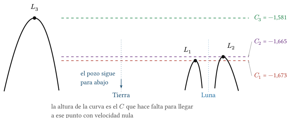
Figura 3: El potencial de Jacobi a lo largo de la línea Tierra-Luna, que es el diagrama de energía del módulo 5 aplicado a este problema. Lo que hay que sacar del dibujo es cómo se lee: la nave tiene un C fijo, que se dibuja como una recta horizontal, y sólo puede estar donde esa recta queda por encima de la curva. Los tres máximos son L_1 , L_2 y L_3 — y que sean máximos es la razón de que los tres sean inestables. La ventana vertical es angosta a propósito: mide 0,19 \text{ km}^2/\text{s}^2 de alto, porque las tres alturas que importan están dentro de ese rango y con una ventana que mostrara los dos pozos enteros, C_1 y C_2 quedarían encimadas. Los dos pozos se van por abajo del dibujo, y ahí es donde están la Tierra y la Luna.
