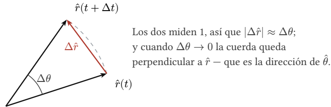
Figura 3: Dos posiciones del mismo versor, separadas \Delta \theta . Como los dos miden 1, la cuerda que los une mide \Delta \theta (en radianes) y, en el límite, es perpendicular a \hat{r} .
