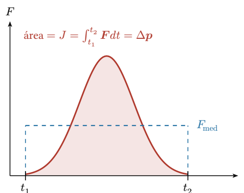
Figura 1: La fuerza de un choque es un pico corto de forma desconocida. El impulso es el área bajo la curva, y esa área es todo lo que hace falta. La fuerza media F_{\text{med}} se define, justamente, como la altura del rectángulo de igual área.
