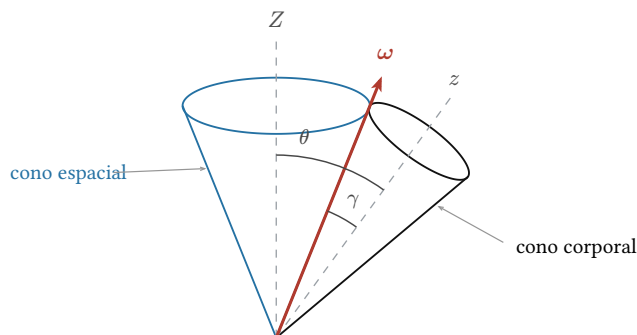
Figura 2: Los dos conos, en el caso de precesión estable —el de los módulos 20 y 21—, donde los dos son circulares. Z es el eje alrededor del cual precesa el cuerpo; z es su eje de simetría; \omega es el eje instantáneo, la generatriz común. El cono corporal está clavado al cuerpo y rueda sobre el espacial, que está clavado al espacio.
