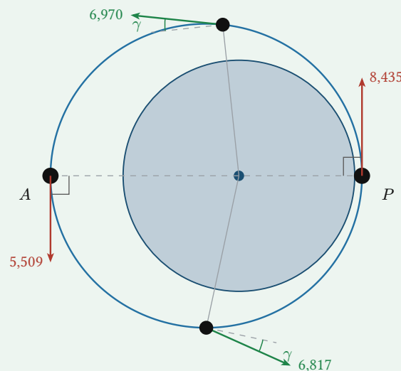
Figura 3: El satélite del ejercicio, redibujado con los datos de la figura de la cátedra. En los ápsides v es perpendicular al radio; en las dos posiciones intermedias forma un ángulo \gamma con esa perpendicular. Velocidades en km/s.
