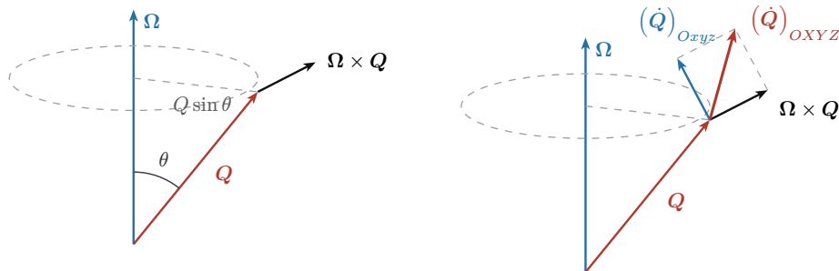
Figura 3: La ec. (10), en sus dos casos. Izquierda: si Q está clavado al sistema que rota, su punta recorre un círculo de radio Q \sin \theta y su derivada es la velocidad de esa punta, \Omega \times Q , tangente al círculo y de módulo \Omega Q \sin \theta . Derecha: si además Q cambia dentro del sistema, las dos contribuciones se suman como vectores.
