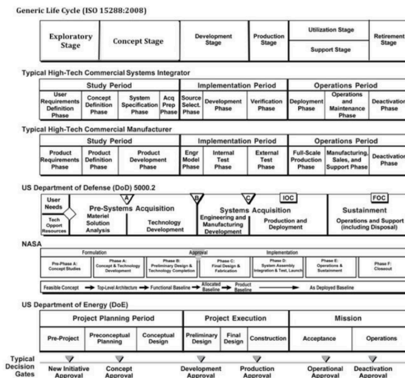
Figura 7: Seis modelos de ciclo de vida lado a lado —ISO 15288, integrador comercial típico, fabricante comercial típico, DoD, NASA y DoE— con sus fases y sus baselines marcados (diapositiva 85).
