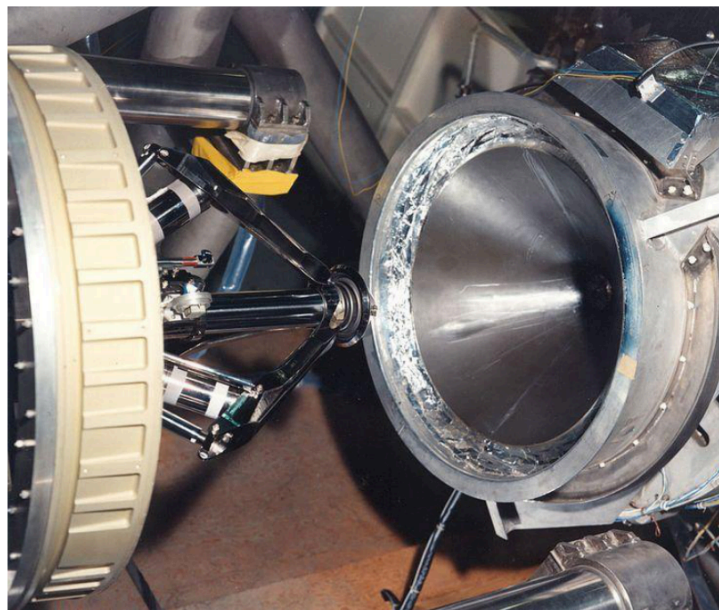
Figura 4: El sistema de acoplamiento (docking) real del Programa Apollo — la interfaz física entre el Módulo de Comando/Servicio y el Módulo Lunar.
