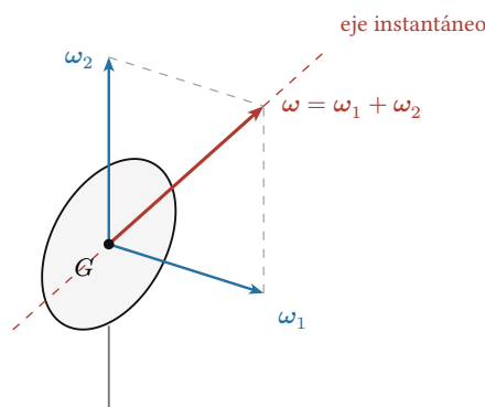
Figura 1: El disco de la horquilla, ya visto en el módulo 18 (allá, para hallar \omega ; acá, para hallar \mathbf{H}_G ). Los ejes \hat{i}, \hat{j}, \hat{k} , clavados a la horquilla, son en todo instante ejes principales del disco: \hat{k} es su eje de simetría y \hat{i}, \hat{j} son diámetros.
