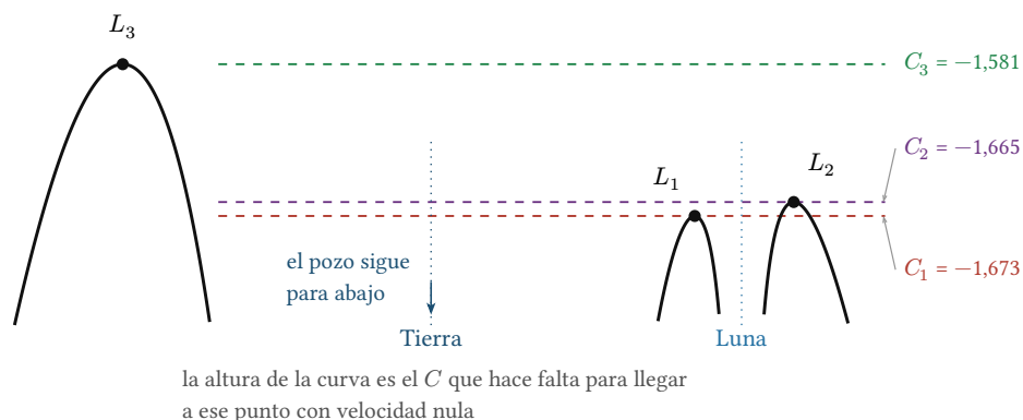
Figura 3: El potencial de Jacobi a lo largo de la línea Tierra-Luna, que es el diagrama de energía del módulo 6 aplicado a este problema. Lo que hay que sacar del dibujo es cómo se lee: la nave tiene un C fijo, que se dibuja como una recta horizontal, y sólo puede estar donde esa recta queda por encima de la curva. Los tres máximos son L_1 , L_2 y L_3 — y que sean máximos es la razón de que los tres sean inestables. La ventana vertical es angosta a propósito: mide 0,19 \text{ km}^2/\text{s}^2 de alto, porque las tres alturas que importan están dentro de ese rango y con una ventana que mostrara los dos pozos enteros, C_1 y C_2 quedarían encimadas. Los dos pozos se van por abajo del dibujo, y ahí es donde están la Tierra y la Luna.
