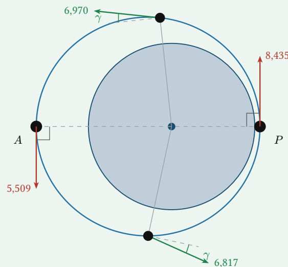
Figura 3: El satélite del ejercicio, redibujado con los datos de la figura de la cátedra. En los ápsides \mathbf{v} es perpendicular al radio; en las dos posiciones intermedias forma un ángulo \gamma con esa perpendicular. Velocidades en km/s.
