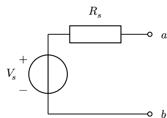
MODELO DE TENSIÓN
