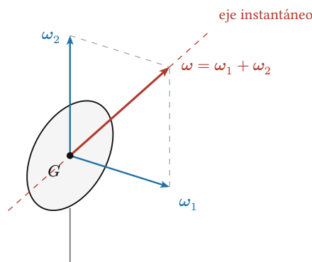
Figura 1: El disco del Problema 2 de la guía: la horquilla gira con \omega_2 alrededor de la vertical y el disco gira con \omega_1 alrededor de su propio eje. Su velocidad angular es la suma de las dos, y la recta que la contiene —punteada— es el eje instantáneo de rotación. Nótese que ese eje no está fijo ni al espacio ni al disco: barre un cono en cada uno.
