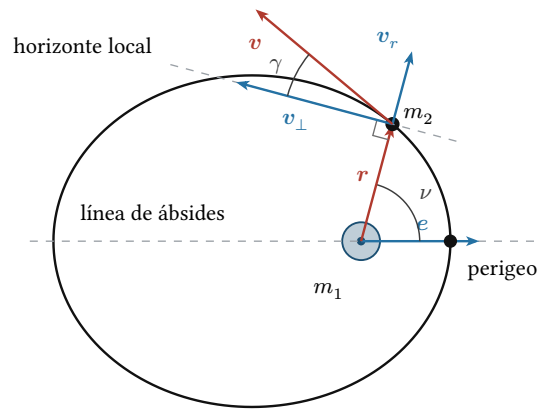
Figura 3: La velocidad en el horizonte local , que es la perpendicular al radio y no la tangente a la órbita: v_{\perp} va sobre el horizonte, v_r sobre el radio, y \gamma es lo que la velocidad se sale del horizonte. Vale para las cuatro cónicas, no sólo para la elipse dibujada.
