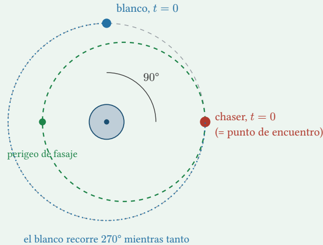
Figura 2: El rendez-vous por fasaje: el chaser baja a una elipse de fasaje tangente en su propio punto de partida —que ahí es el apogeo—, completa una vuelta en tres cuartos del período circular, y llega exactamente cuando el blanco, que mientras tanto recorrió 270^\circ , también llega.
