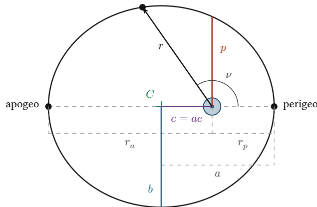
Figura 3: La elipse orbital y todo lo que se le mide. Arriba de la línea de ápsides, lo que se mide desde el foco : el parámetro p , el radio r de un punto cualquiera y su anomalía verdadera \nu . Abajo, lo que se mide desde el centro : los semiejes a y b , y las dos distancias de ápside. El cuerpo central está en el foco F , nunca en el centro C — y la distancia entre los dos es exactamente ae .
