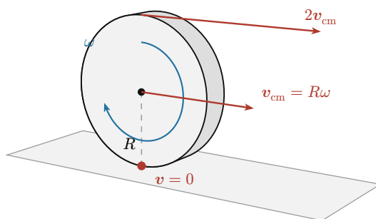
Figura 4: Una rueda que rueda sin deslizar. El centro avanza con v_{\text{cm}} = R\omega ; el punto de contacto está quieto en ese instante y el de arriba va a 2v_{\text{cm}} . La energía cinética es la del centro de masa más la de la rotación alrededor de él. Como en S&Z, pág. 310–313.
