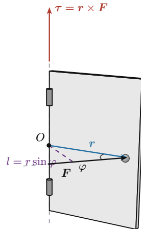
Figura 3: La puerta, en perspectiva. La fuerza F en el picaporte, a r del eje de las bisagras, hace un torque \tau = r \times F que apunta sobre ese eje (hacia arriba, por la mano derecha), de módulo Fl , con l = r \sin \varphi el brazo de palanca: la distancia de O a la recta de acción de F . La misma fuerza cerca de las bisagras tiene r chico y no abre nada. La idea es la de S&Z pág. 305.
