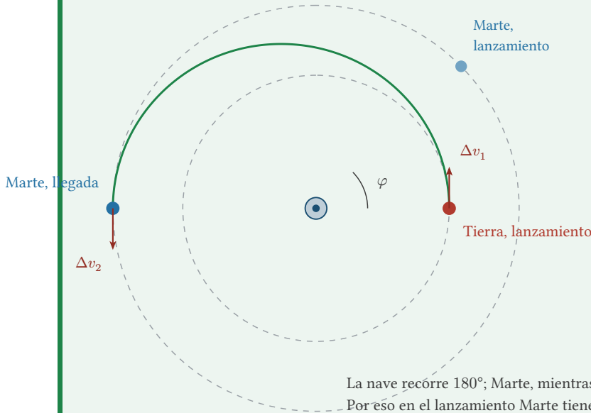
Figura 1: La transferencia de Hohmann Tierra-Marte (a escala aproximada de radios). La nave recorre 180° en 258,8 días; Marte, mientras tanto, recorre 135,6° de su propia órbita — por eso en el lanzamiento tiene que estar apenas 44,4° adelante de la Tierra, no en el punto de encuentro.
