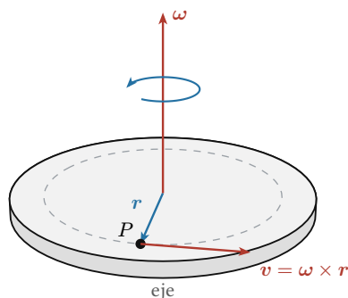
Figura 1: Un rígido que gira alrededor de un eje fijo. La velocidad angular es un vector sobre el eje: con los dedos de la mano derecha acompañando el giro, el pulgar marca \omega . Cada punto P recorre un círculo alrededor del eje con v = \omega \times r , tangente, de módulo \omega r , con r la distancia al eje. Como la S&Z Fig. 9.5, pág. 276.
