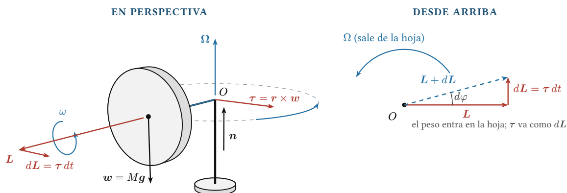
Figura 6: El giróscopo apoyado en un pivote. En perspectiva: el peso w = Mg , en el centro de masa, hace respecto del pivote O un torque \tau = r \times w horizontal y perpendicular al eje. dL = \tau dt va para el mismo lado, así que la punta de L se corre de costado y el eje gira alrededor del poste con \Omega . Desde arriba: ese dL perpendicular hace girar el eje un ángulo d\varphi sin cambiarle el largo. Redibujada de S&Z Figs. 10.34 y 10.35, pág. 323–324.
