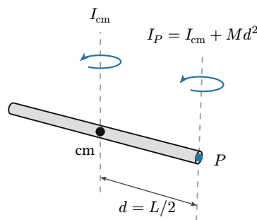
Figura 2: Dos ejes paralelos: uno por el centro de masa y otro a distancia d . El momento de inercia respecto del segundo es el del primero más Md^2 . Para la varilla, con d = L/2 , da \frac{1}{3}ML^2 : el de la tabla.
