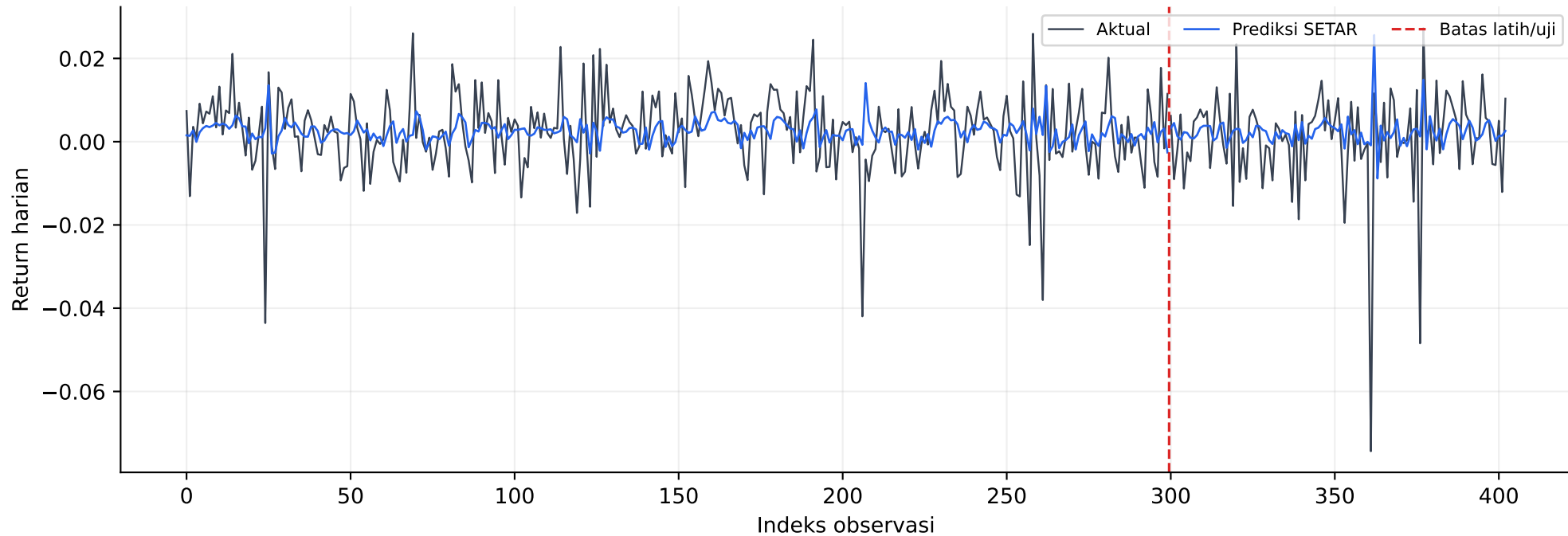
Return aktual dan prediksi SETAR
