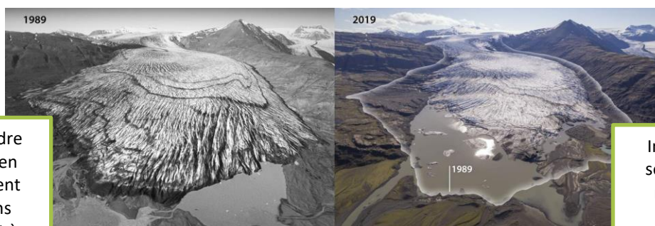
Figure 1 Le glacier Skálafellsjökull en 1989 et en 2019
