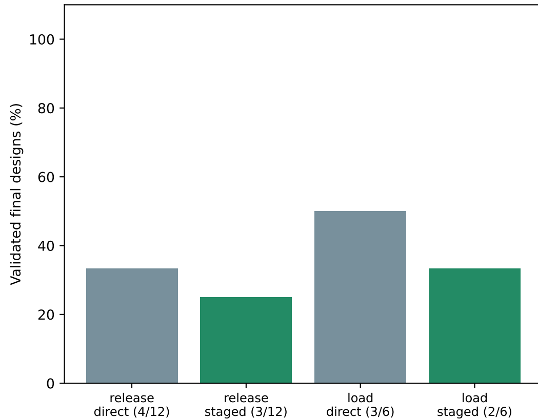
madnlp
