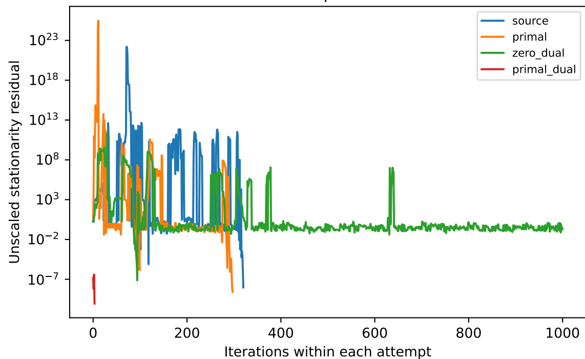
IEEE 300 | load 1.05
