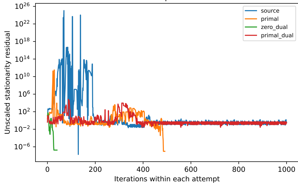
IEEE 300 | load 1.05
