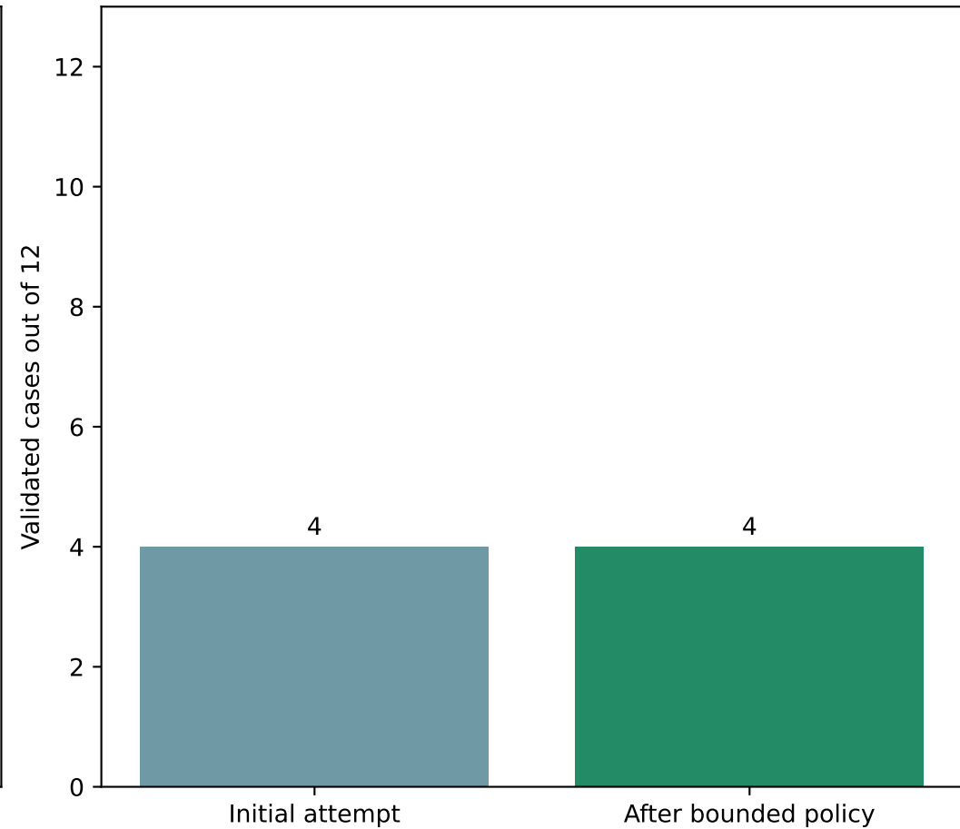
madnlp
