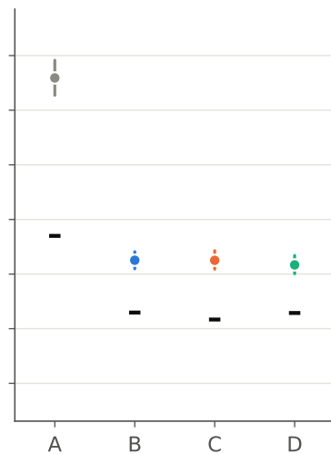
Qwen3 32B
