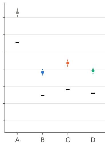
Ministral 3B
