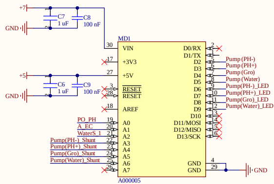
ARDUINO NANO
