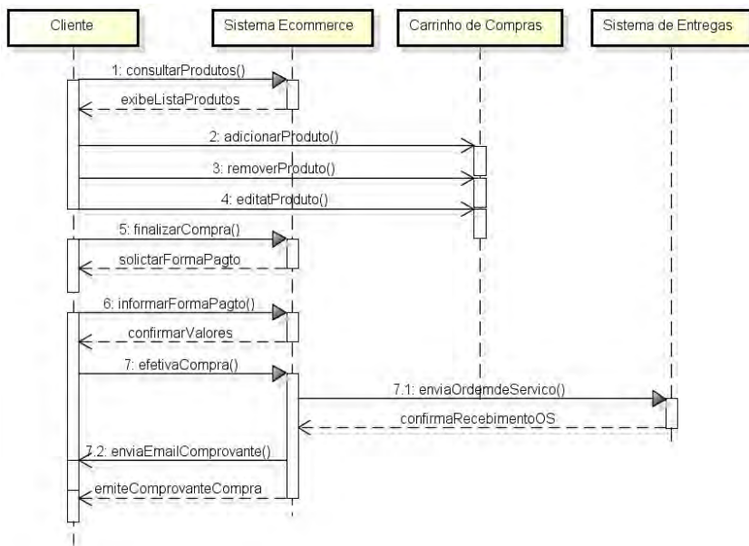
Figura 10.3: Diagrama de Seqüência
