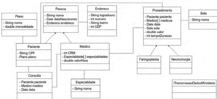
Figura 8.2: Modelagem com atributos
