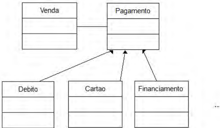
Figura 9.2: Acoplamento fraco
