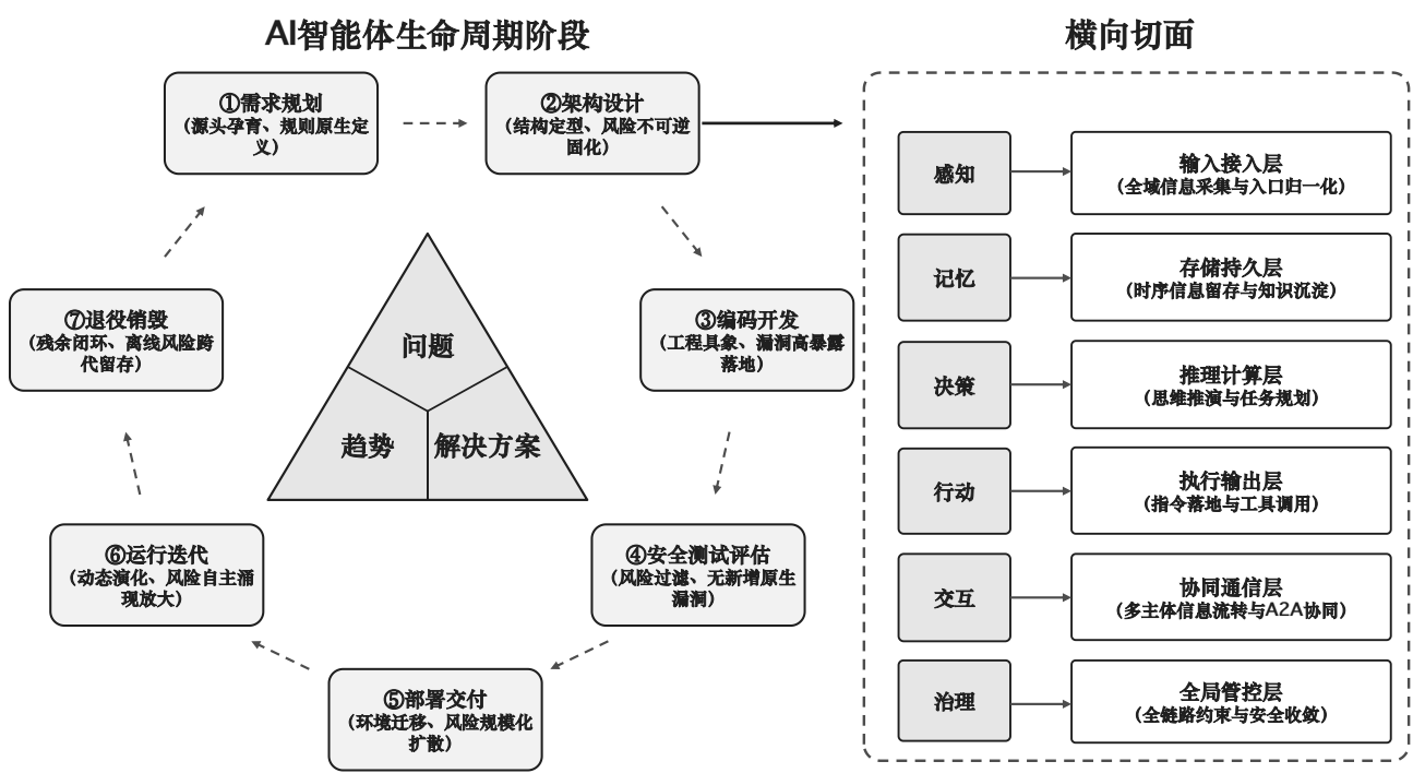
图 1.1: AI 智能体生命周期阶段分析框架，其中包括七大生命周期阶段，每个阶段包括六大业务横切面。
