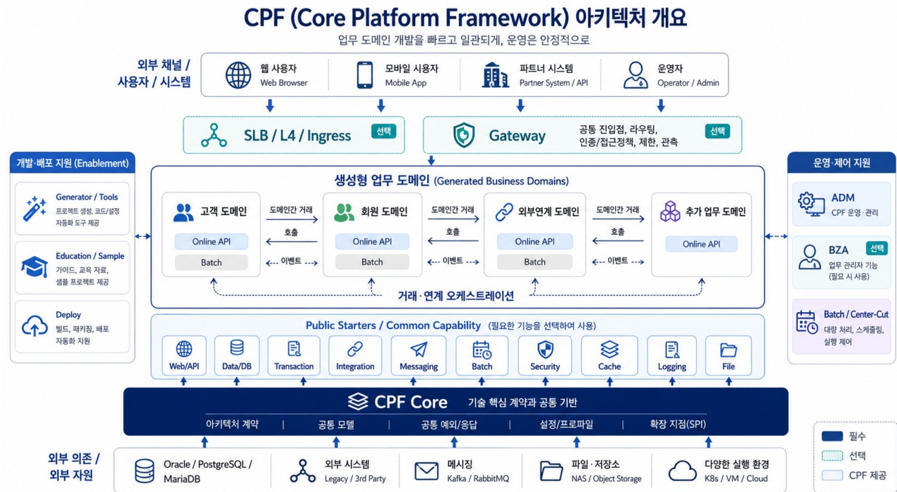
업무 Domain 과 선택 Runtime 의 배치 구조
