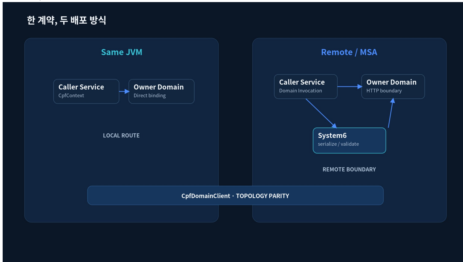
그림 4-1. Split Compare - 이 절의 Owner, 흐름 또는 상태 전이를 한눈에 확인합니다.
