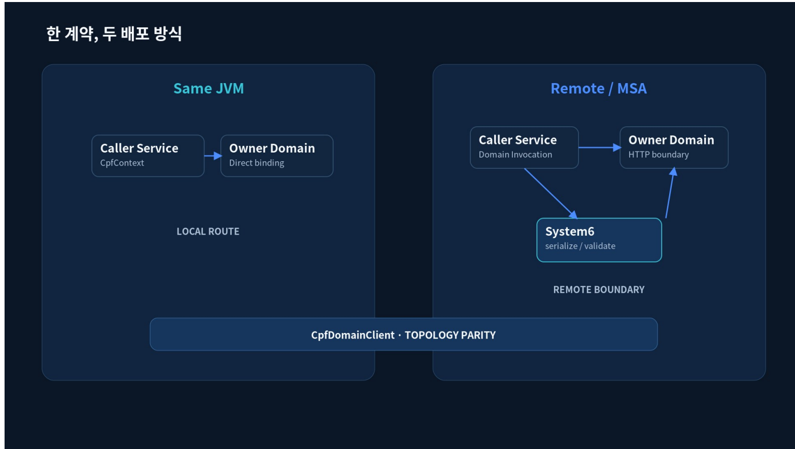
그림 1-1. Split Compare - 이 절의 Owner, 흐름 또는 상태 전이를 한눈에 확인합니다.
