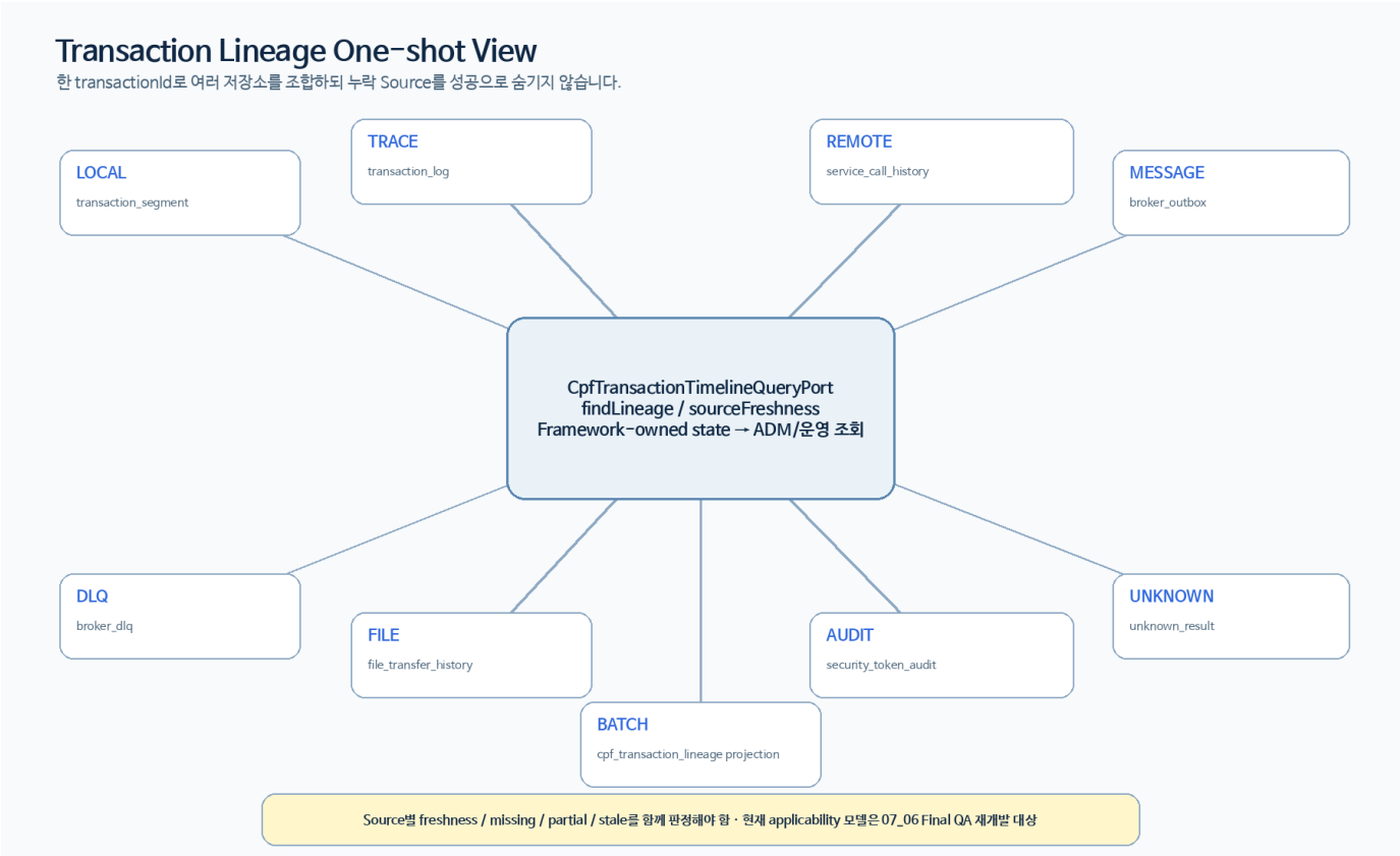
그림 0-1. transactionId one-shot lineage와 Source freshness/partial 판단
