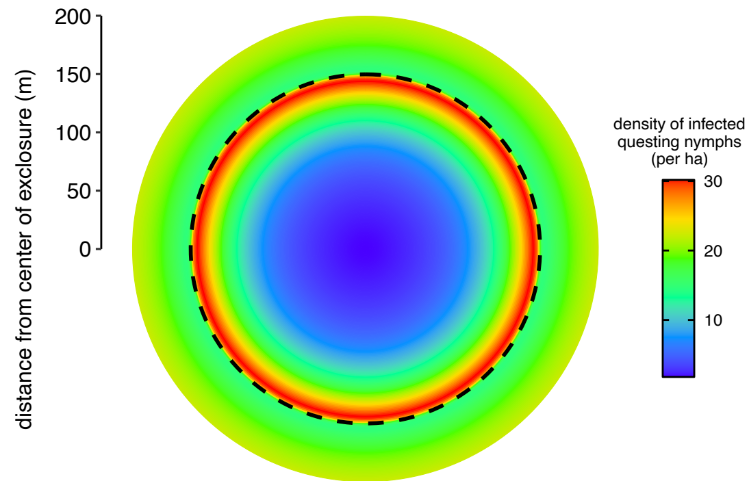
(d) questing tick movement, large enclosure
