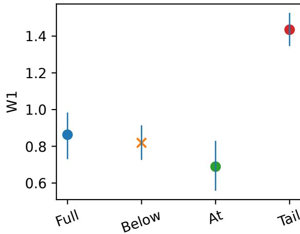
mixture, K=2048
