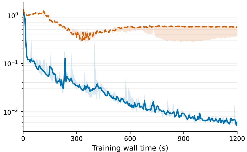
CH6 (order 6)
