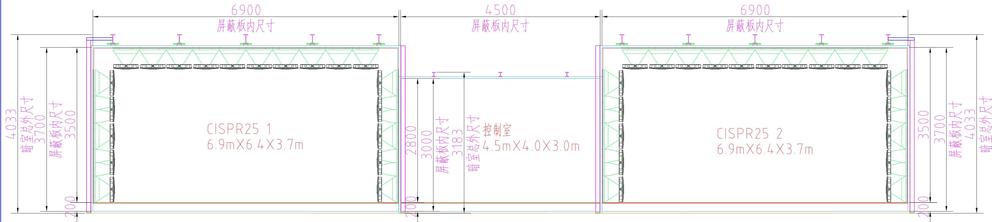
暗室屏蔽室南侧剖立面布局图
