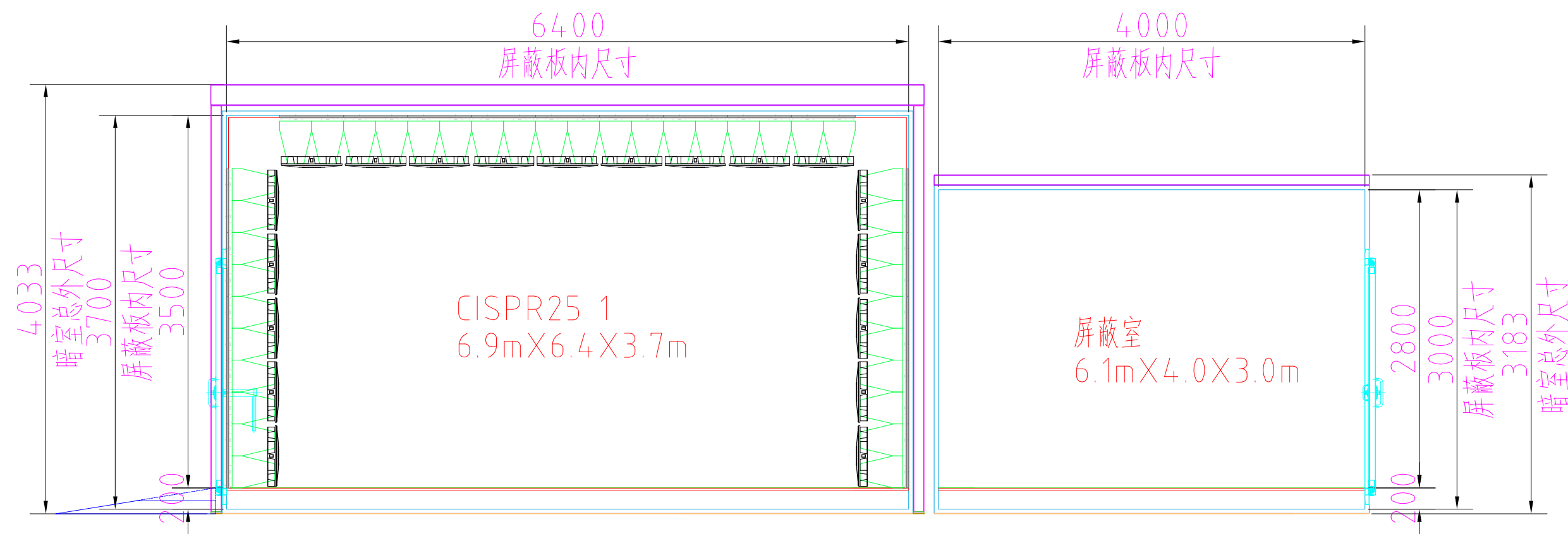
暗室屏蔽室西侧剖立面布局图
