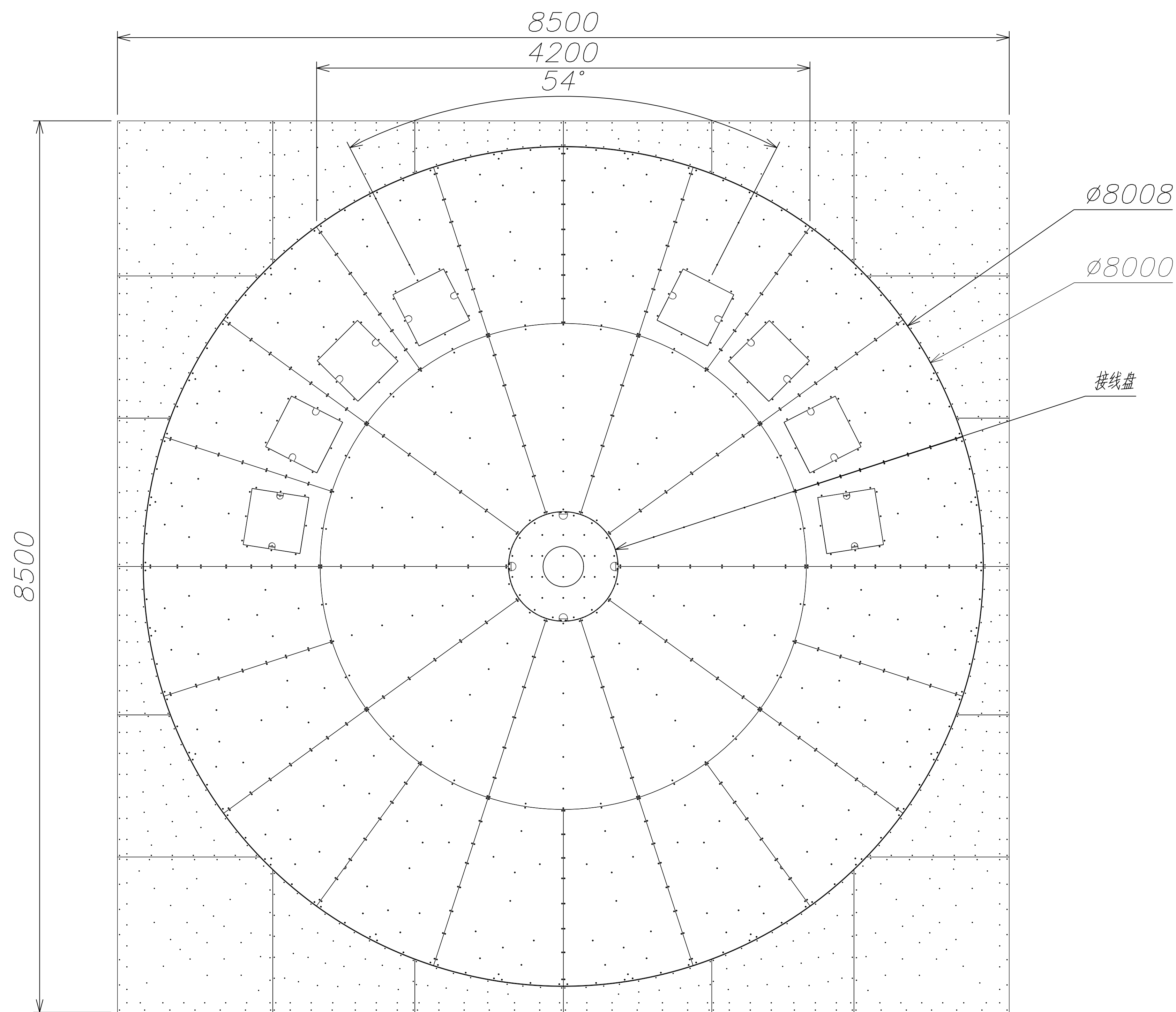
8米转台（内置回转拖链系统）投影
