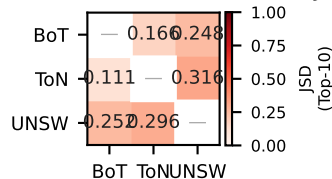
(d) Reconnaissance JSD [Top-10]
