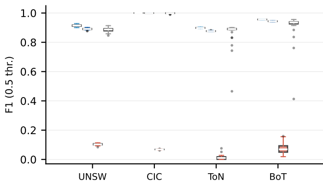
(c) DoS — F1 at default 0.5 threshold
