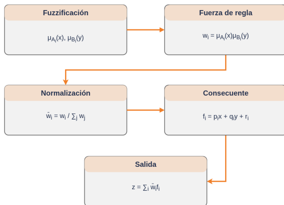
(a) Arquitectura por capas de un modelo ANFIS de dos entradas.
