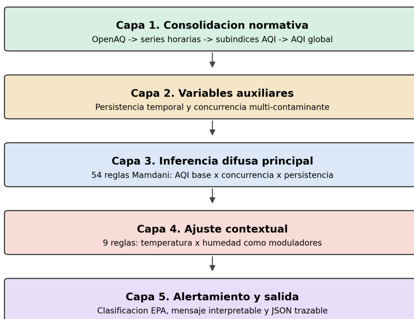
Figura 8. Arquitectura funcional implementada del módulo AQRisk. Elaboración propia.
