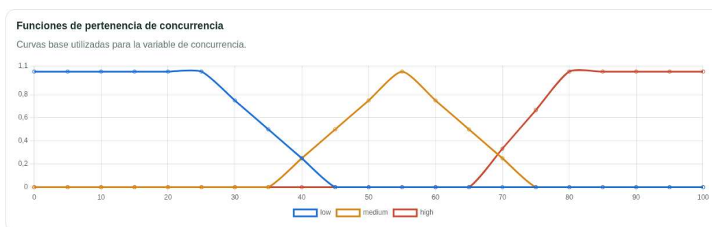
Figura 17. Funciones de pertenencia de concurrencia para la corrida real de Parque O'Higgins . La visualización muestra cómo el artefacto representa la coexistencia efectiva de contaminantes soportados y la incorpora como variable auxiliar en la inferencia principal. Elaboración propia.
