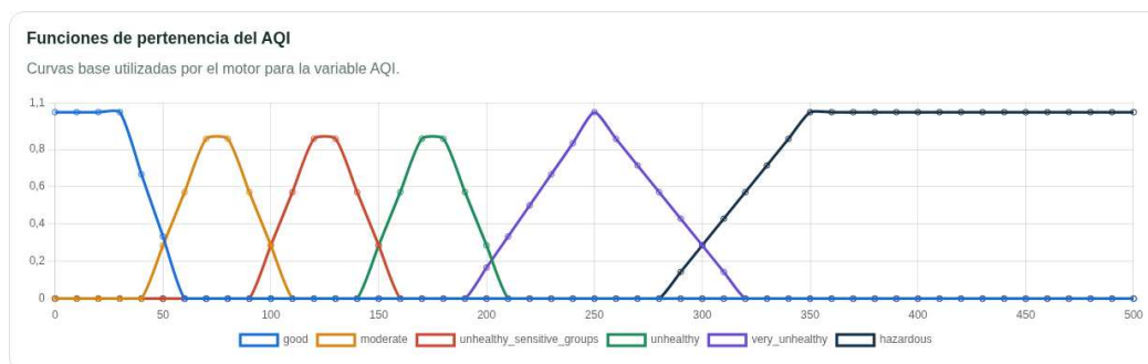
Figura 16. Funciones de pertenencia del AQI para la corrida real de Parque O'Higgins . La figura sitúa el AQI consolidado dentro de las categorías lingüísticas del antecedente normativo y ayuda a justificar por qué el episodio queda ubicado en una zona moderada del sistema difuso. Elaboración propia.
