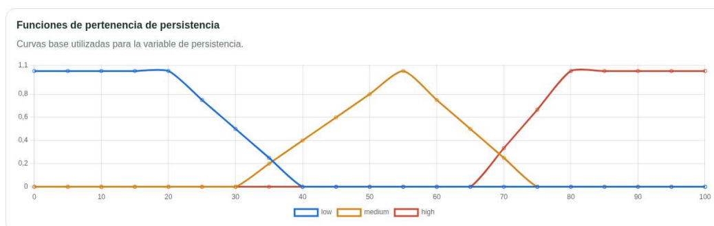
Figura 18. Funciones de pertenencia de persistencia para la corrida real de SAN BORJA . La captura muestra cómo la continuidad temporal del episodio se traduce a términos lingüísticos antes de combinarse con el AQI y la concurrencia en la base principal de reglas. Elaboración propia.
