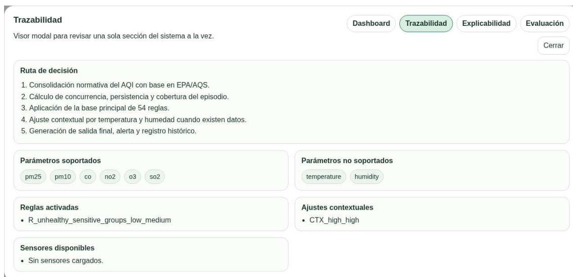
Figura 12. Modal de Trazabilidad para el escenario controlado urban_escalation . La captura muestra soporte completo de contaminantes criterio y un ajuste contextual activo, por lo que complementa la evidencia real con un caso de referencia donde el sistema recorre toda la secuencia prevista por el diseño. Elaboración propia.
