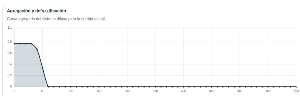
Figura 14. Agregación y defuzzificación de la corrida real de Hospital General de México . La superficie agregada y la puntuación resultante muestran cómo el motor Mamdani transforma la evidencia normativa y auxiliar en una salida crisp sin perder interpretabilidad del proceso intermedio. Elaboración propia.
