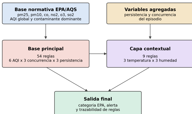
Estructura de decision del modulo IA
