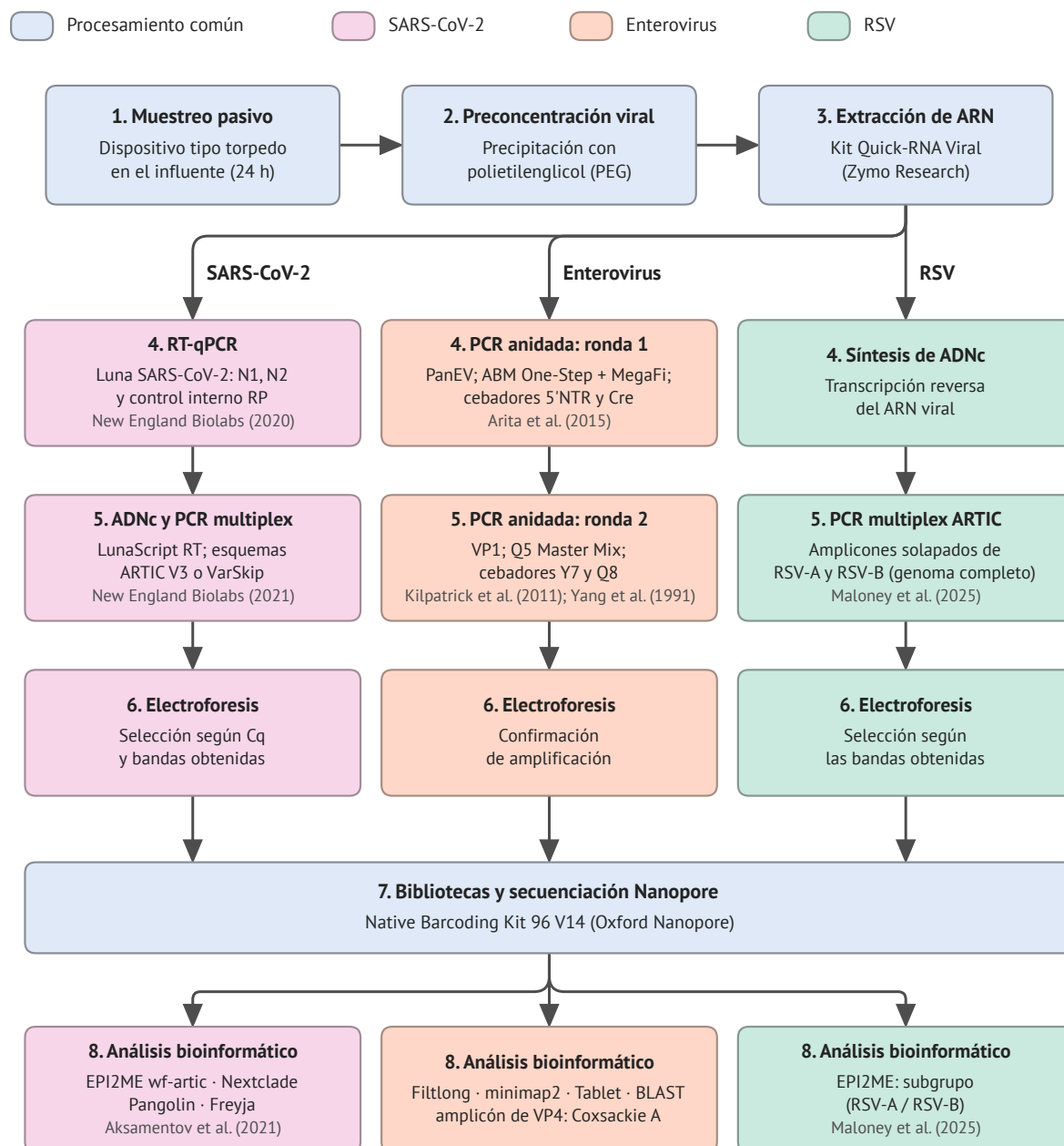
Figura 5. Flujo de trabajo para la detección y caracterización de SARS-CoV-2, enterovirus y RSV. En celeste, las etapas comunes a los tres virus; en rosa, naranja y verde, las etapas específicas de SARS-CoV-2, enterovirus y RSV, respectivamente.
