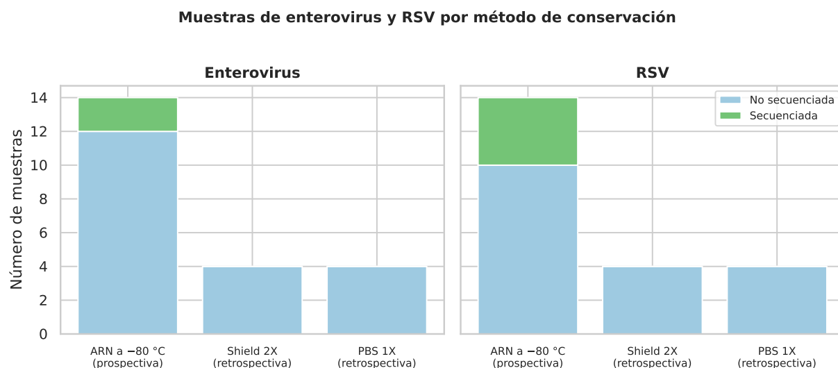
Figura 11. Muestras de enterovirus y RSV según el método de conservación. Las muestras prospectivas, cuyo ARN extraído se almacenó a -80^{\circ}\text{C} , concentraron la totalidad de las secuenciaciones; las muestras retrospectivas conservadas en Shield 2X y en PBS 1X no rindieron secuencia.
