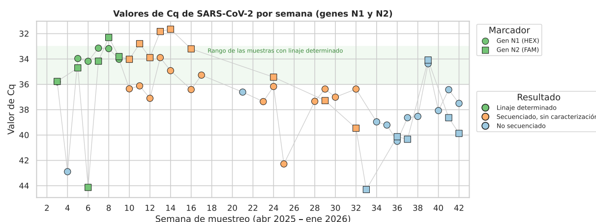
Figura 8. Valores de Cq de SARS-CoV-2 por semana para los genes N1 (HEX) y N2 (FAM). El eje vertical está invertido, de modo que los valores de Cq más bajos, que corresponden a mayor carga viral, aparecen en la parte superior. El color indica el resultado de la secuenciación; la banda verde señala el rango de Cq de las muestras con linaje determinado.
