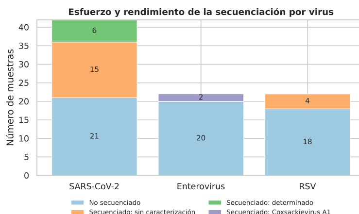
Figura 7. Esfuerzo y rendimiento de la secuenciación por virus. Las barras muestran el número de muestras no secuenciadas, secuenciadas sin caracterización y secuenciadas con caracterización (Coxsackievirus A1 en el caso de enterovirus ).
