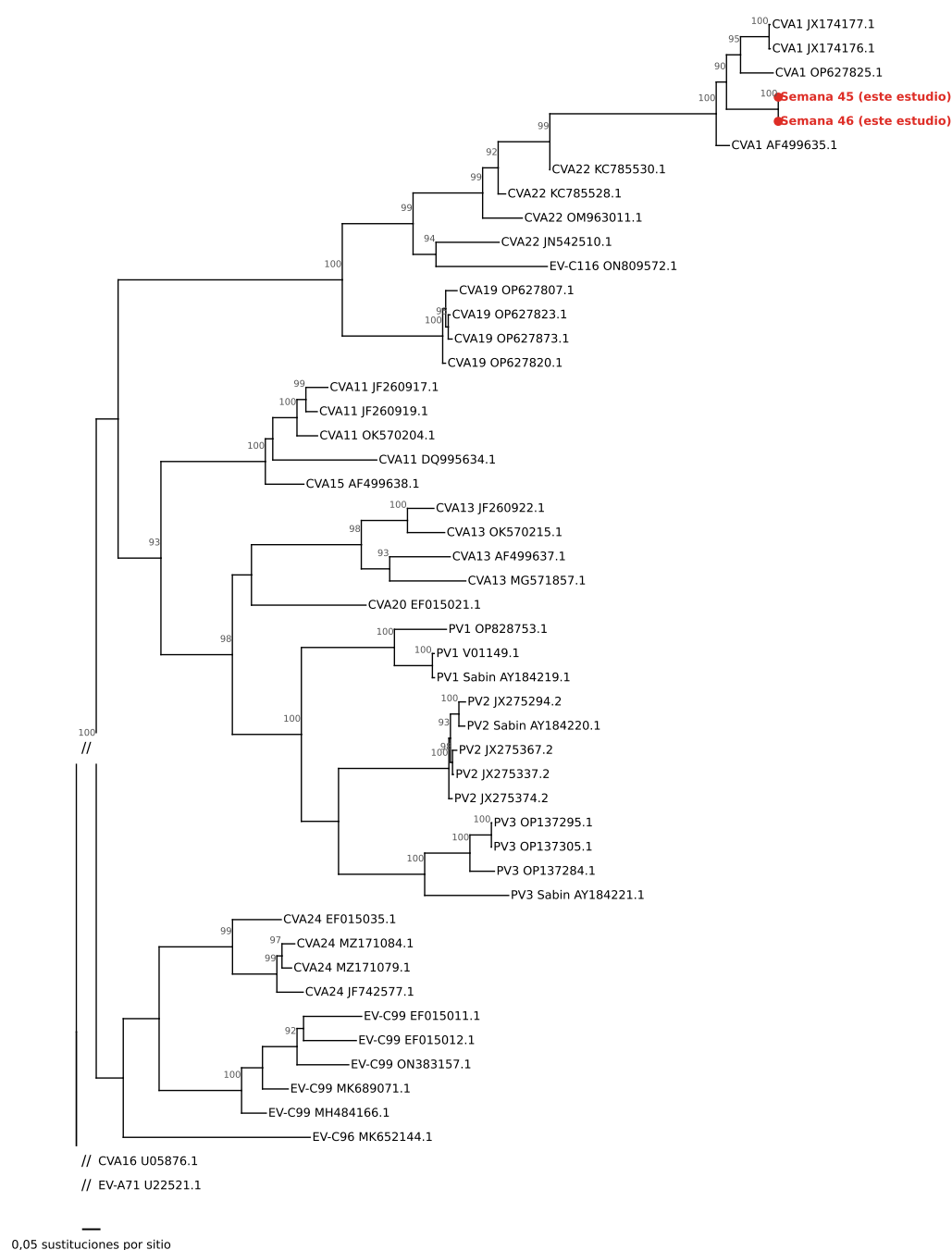
Figura 10. Árbol de máxima verosimilitud de la región VP1 (1094 pb) de enterovirus de la especie C, con enterovirus A como grupo externo. En rojo, los consensos de las semanas 45 y 46. Los números indican el apoyo de bootstrap ultrarrápido ( \geq 90 ). Las ramas marcadas con // se acortaron en el dibujo.
