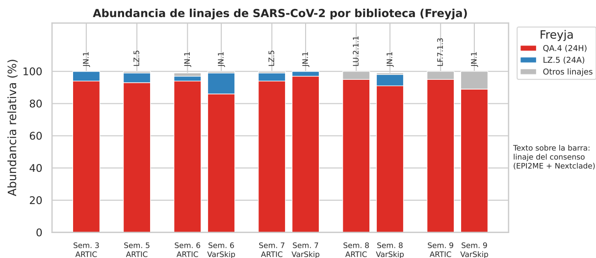
Figura 9. Abundancia relativa de linajes de SARS-CoV-2 estimada con Freyja en las diez bibliotecas de las semanas 3 a 9. Sobre cada barra se indica el linaje asignado al consenso con Nextclade.
