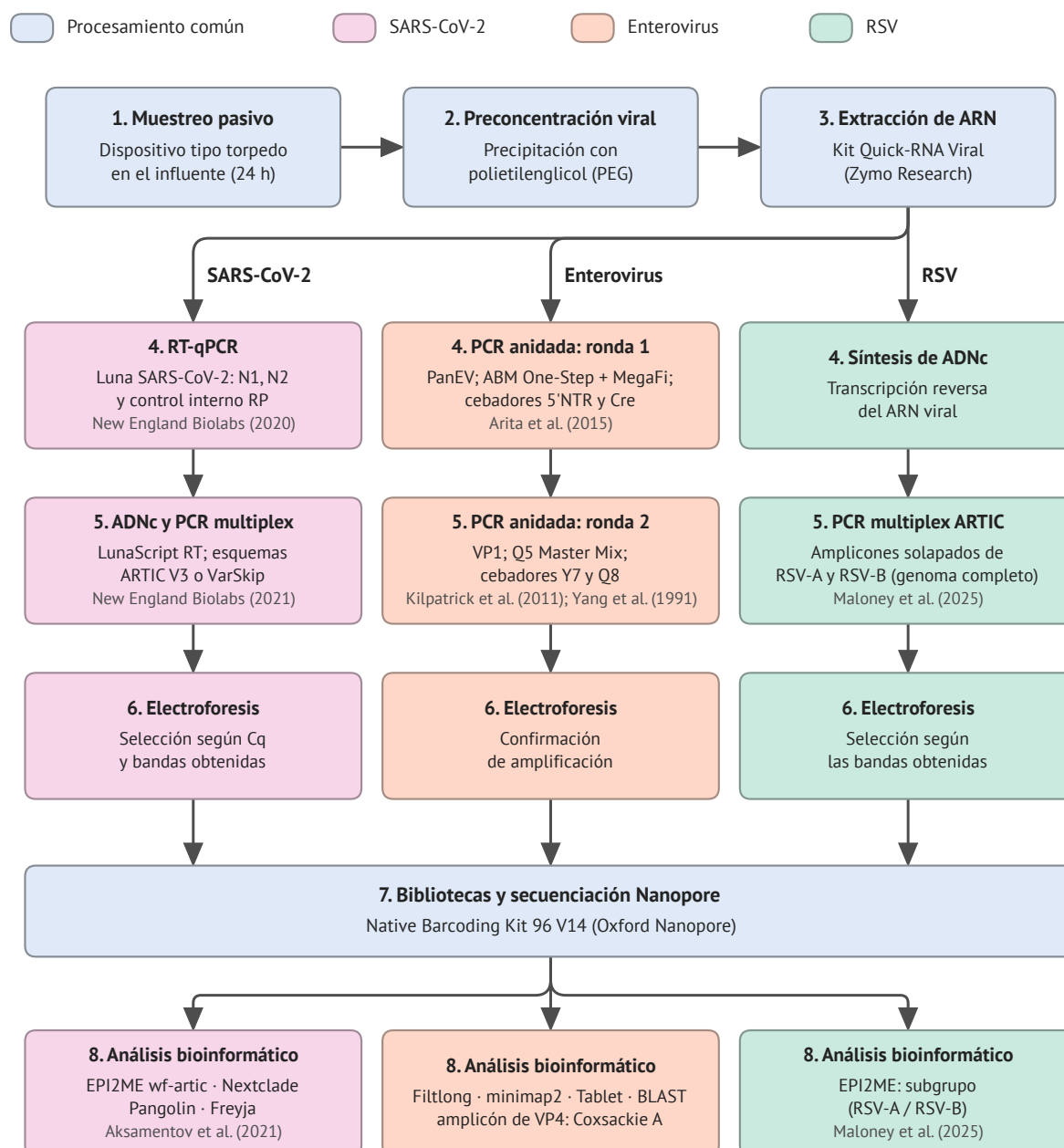
Figura 5. Flujo de trabajo para la detección y caracterización de SARS-CoV-2, enterovirus y RSV. En celeste, las etapas comunes a los tres virus; en rosa, naranja y verde, las etapas específicas de SARS-CoV-2, enterovirus y RSV, respectivamente.
