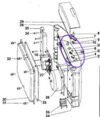
Boutons poussoirs et sélecteurs
