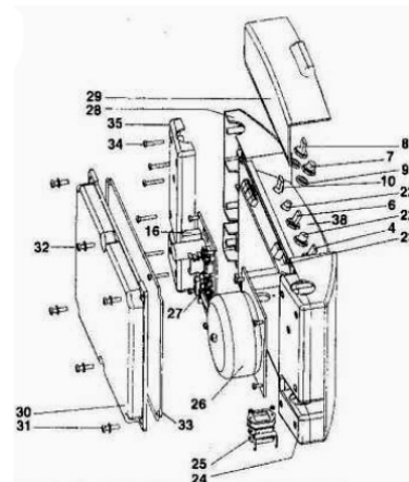
Boutons poussoirs et sélecteurs
