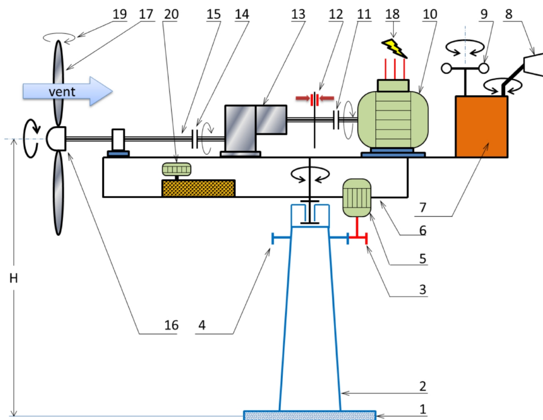
Figure 3: Schéma cinématique "détaillé"
