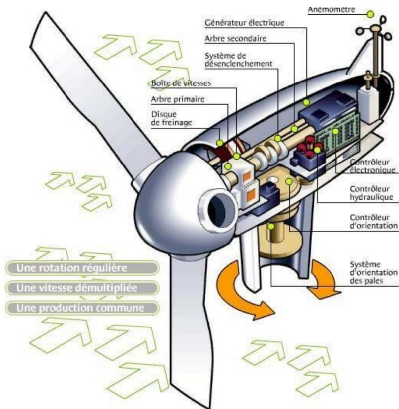
Figure 2: Schéma "simplifié de la nacelle"
