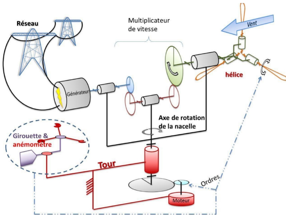
Figure 1: Schéma cinétique de l'éolienne
