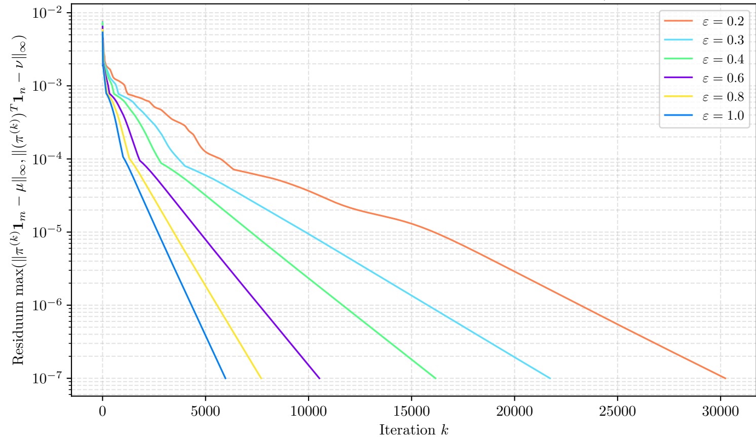
Konvergenzverlauf des Sinkhorn-Algorithmus ( n = 256, m = 256 ) mit Seed=13
