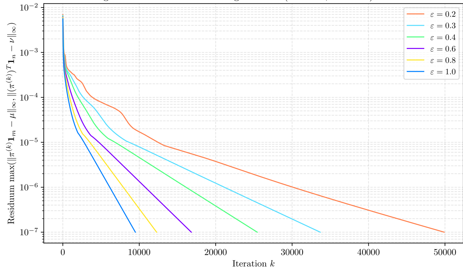
Konvergenzverlauf des Sinkhorn-Algorithmus ( n = 256, m = 256 ) mit Seed=39
