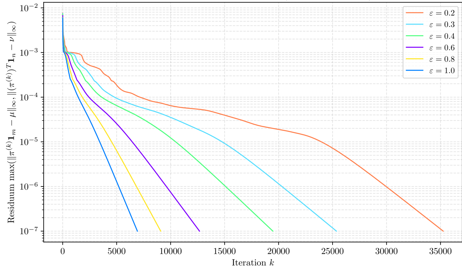
Konvergenzverlauf des Sinkhorn-Algorithmus ( n = 256, m = 256 ) mit Seed=74
